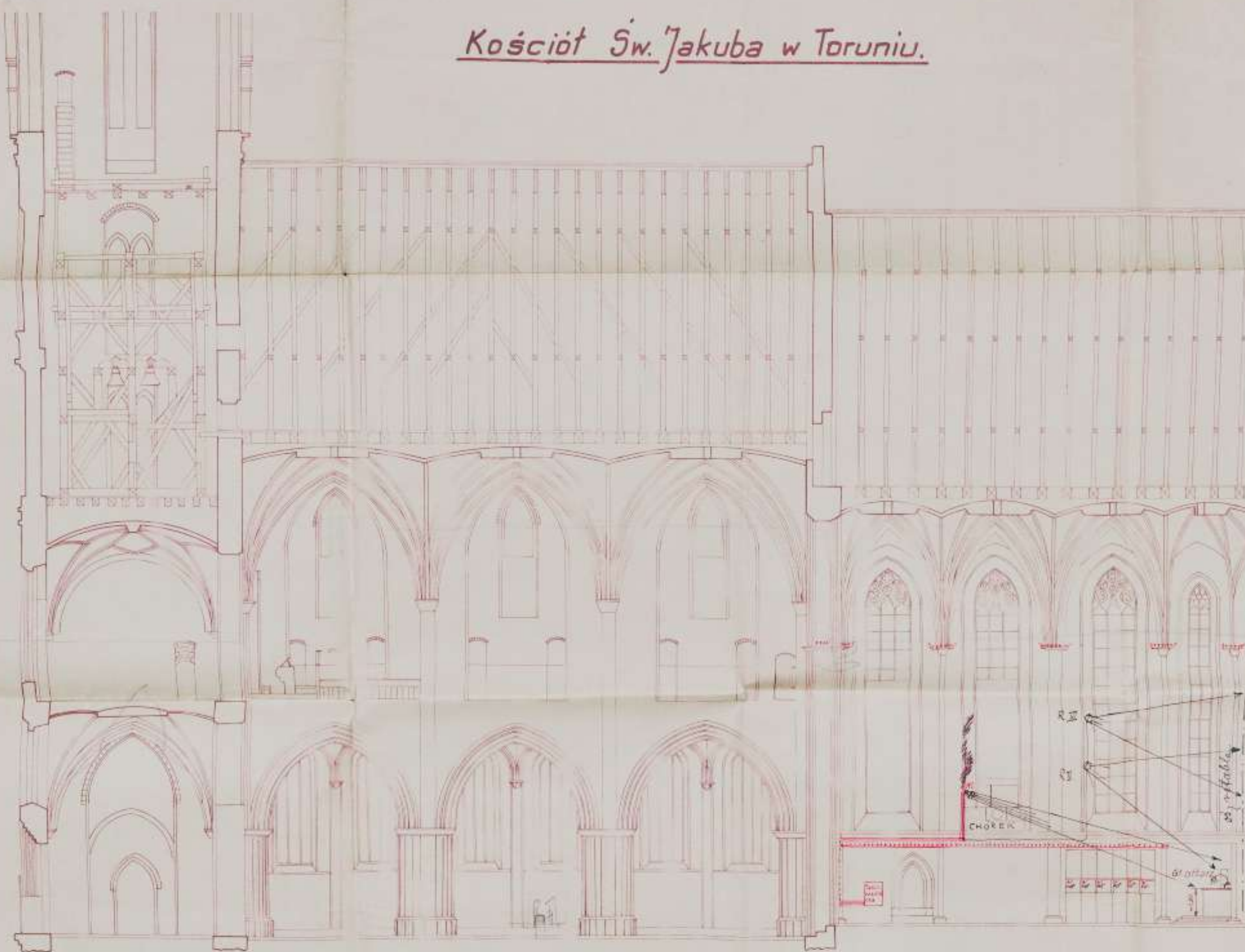
Przekrój podłużny skala 1:100
